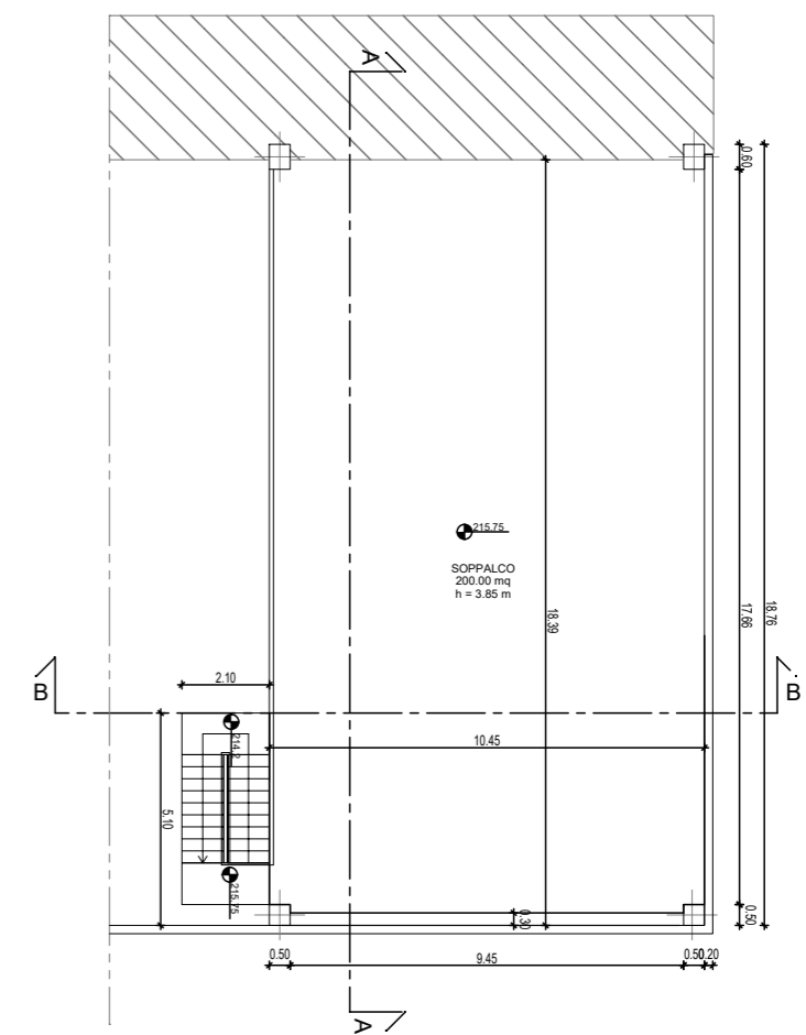
PIANTA SOPPALCO
